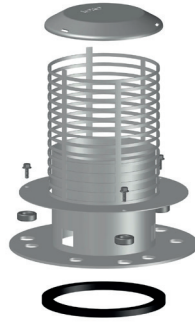
VARIOFIT Retentionseinheit 210 mm Siebkorb 14510.070X 14510.100X 14510.125X
