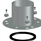
VARIOFIT Notentwässerungseinheit ohne Siebkorb 14709.070X 14709.100X 14709.125X
