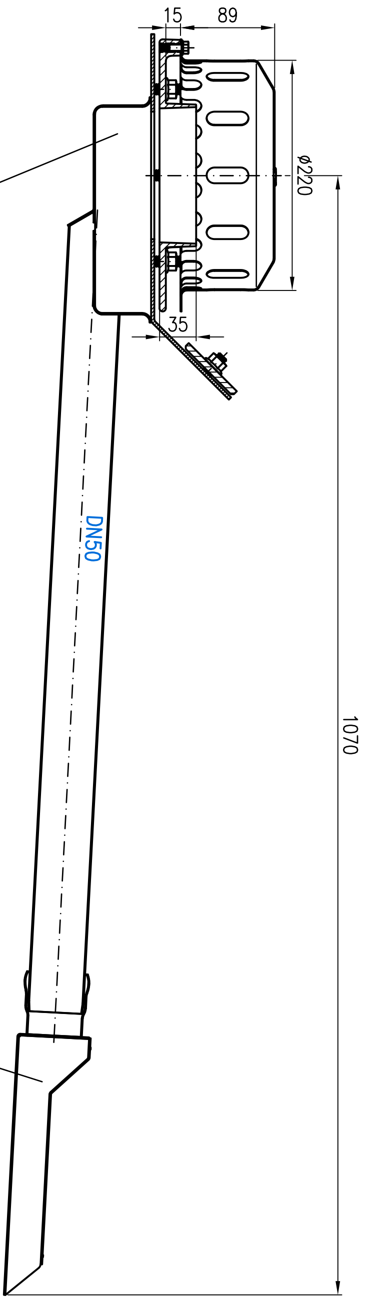
RAINSTAR-Notablauf DN50 EDV-Art.Nr. 01371.050X
