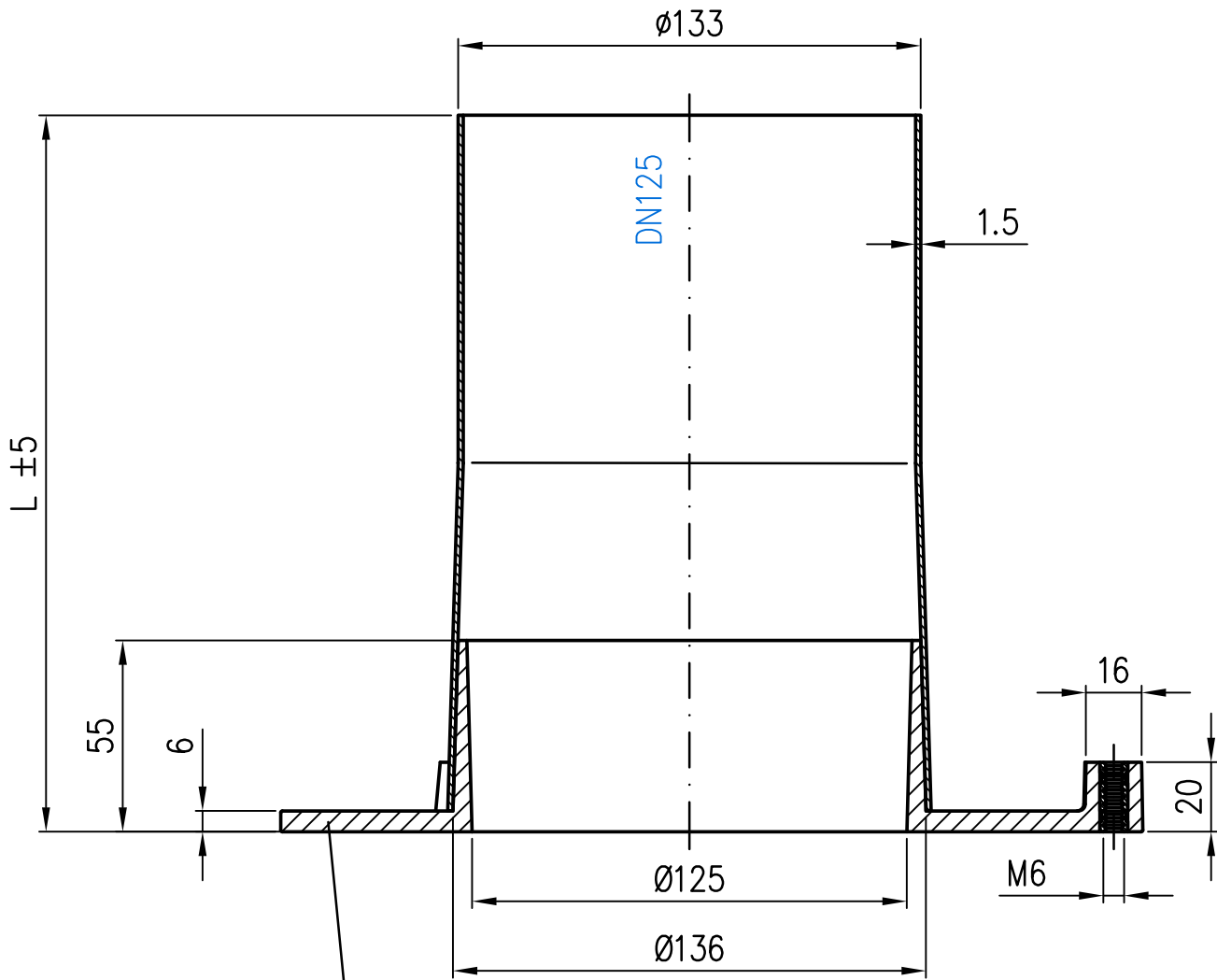
Losflansch EDV-Art.Nr. 21906.070X
