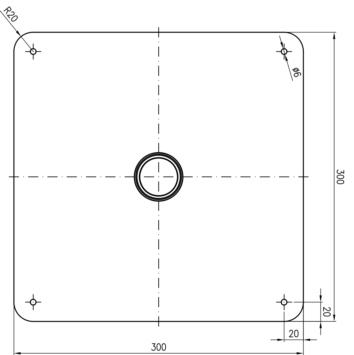
Brennschablone Zchnng.Nr. S903087
