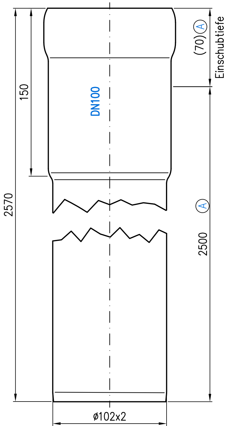
Rohrende leicht eingezogen
