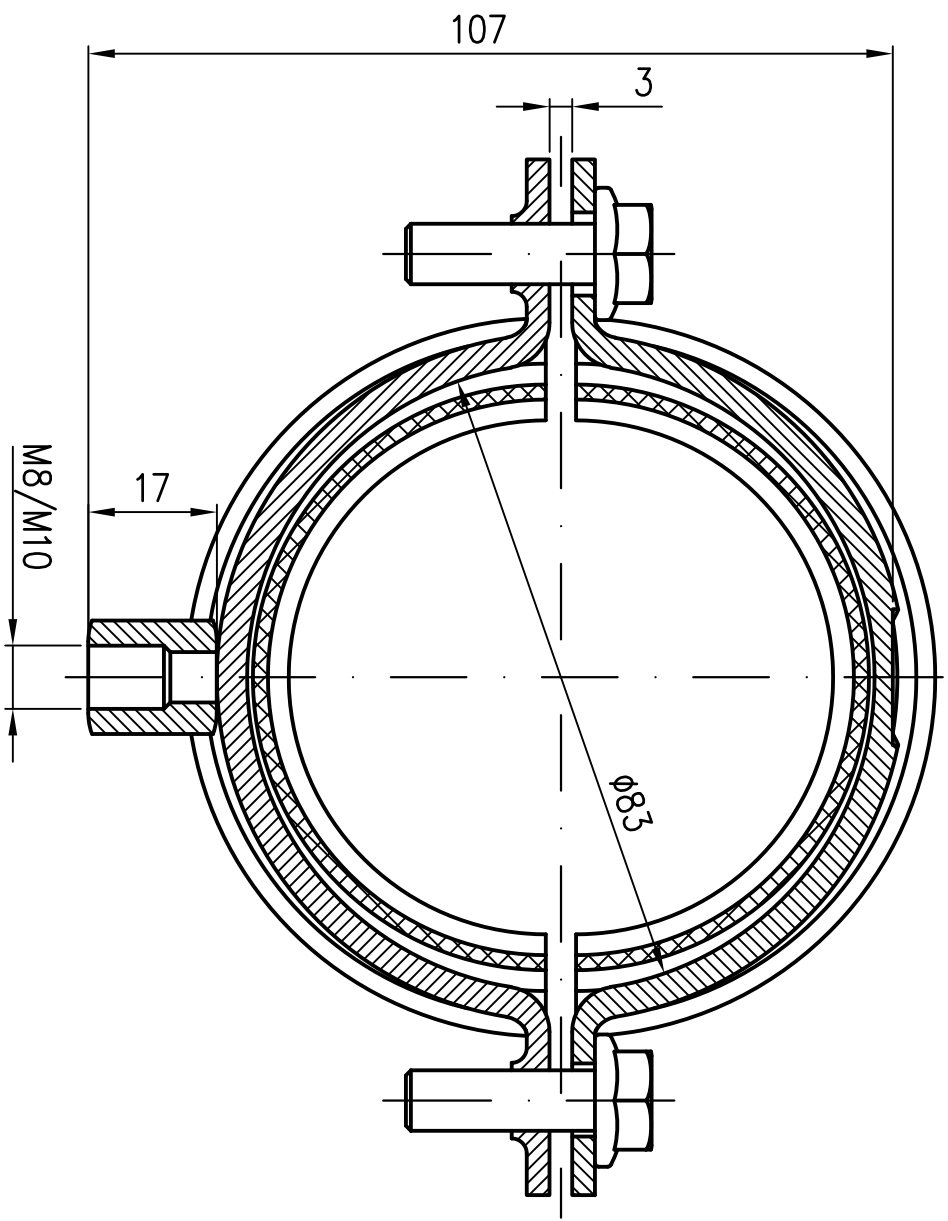
SCHNITT A-A
