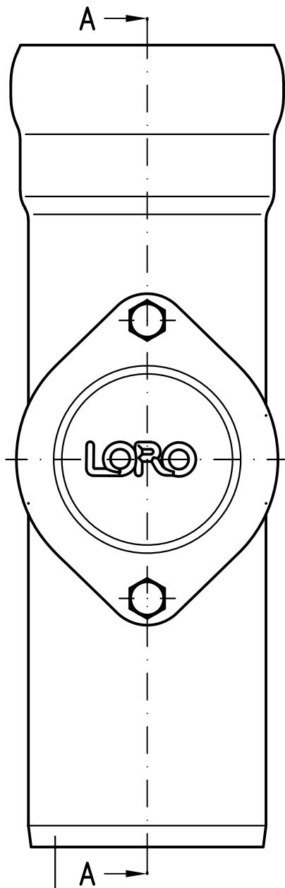
Rohr DN80 Zchnng.Nr. S901064 B
